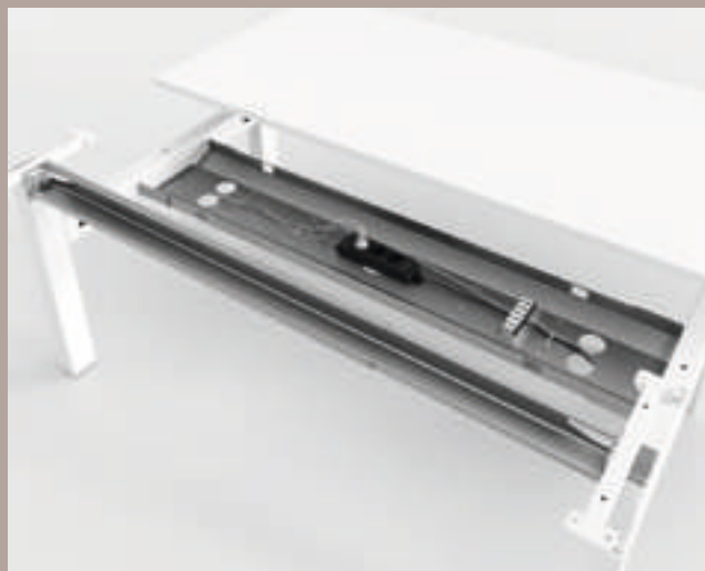
Canalizzazione per tavoli a due scrivanie contrapposte Wire management for bench desks
