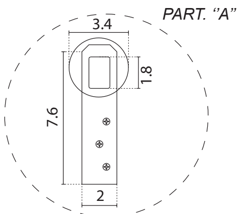
PARTICOLARE MONTAGGIO FISCHER / particularly fitting fischer
