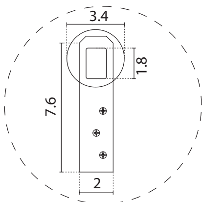
PARTICOLARE MONTAGGIO FISCHER / particularly fitting fischer
