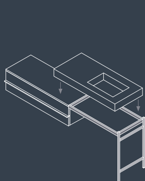
Telaio portaserviette H. 769 a terra L. 776-926 Per piani lavabo integrato H. 120
