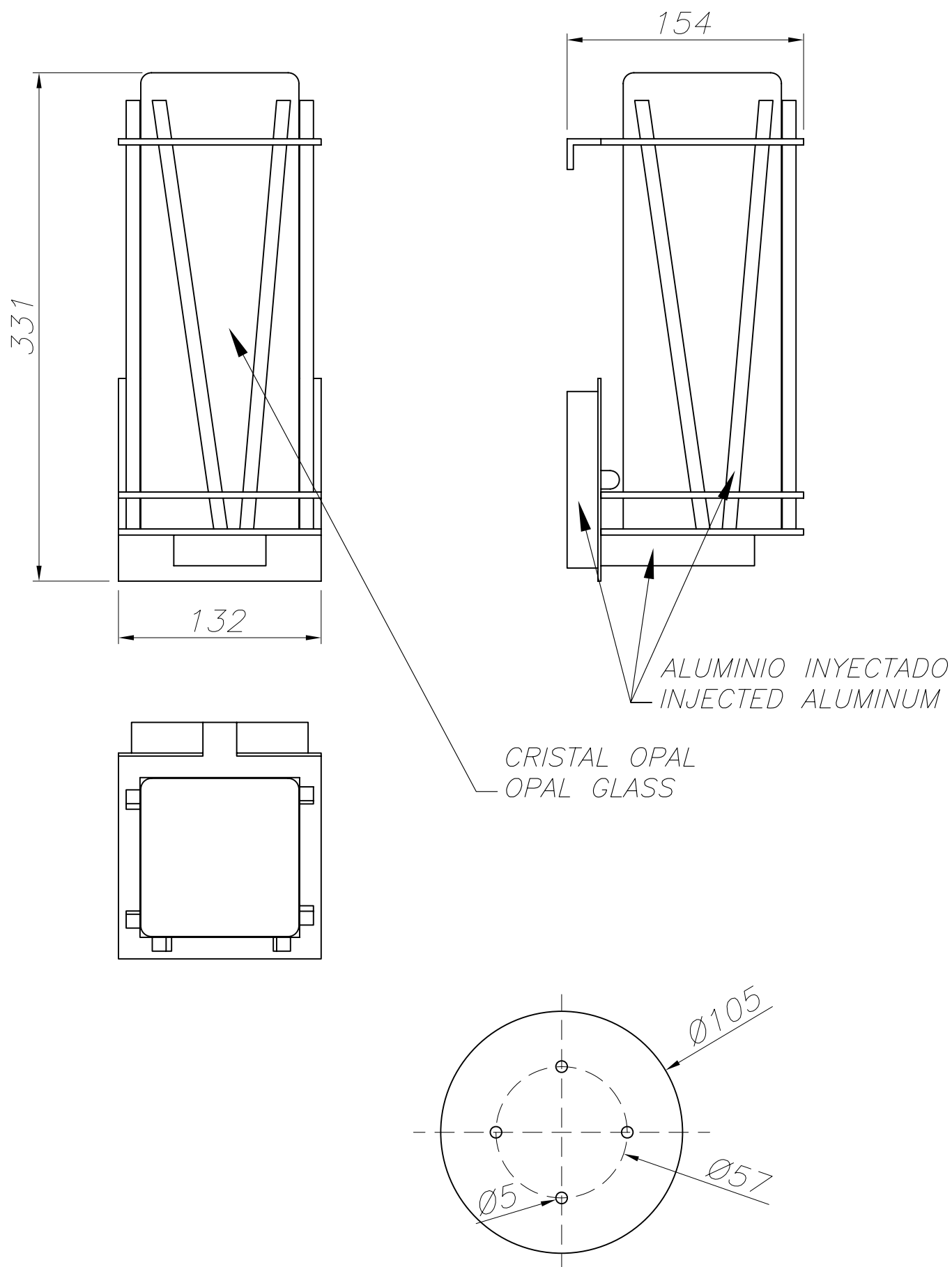
PLANTILLA DE INSTALACIÓN INSTALLATION TEMPLATE
