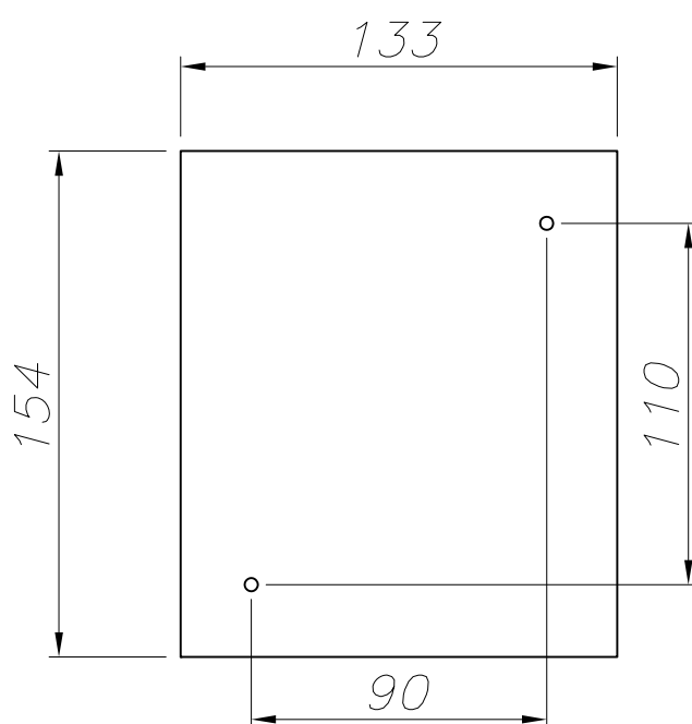
PLANTILLA DE INSTALACIÓN INSTALLATION TEMPLATE
