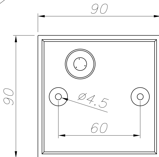
PLANTILLA DE INSTALACIÓN INSTALLATION TEMPLATE
