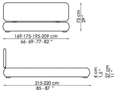
Pad alto
