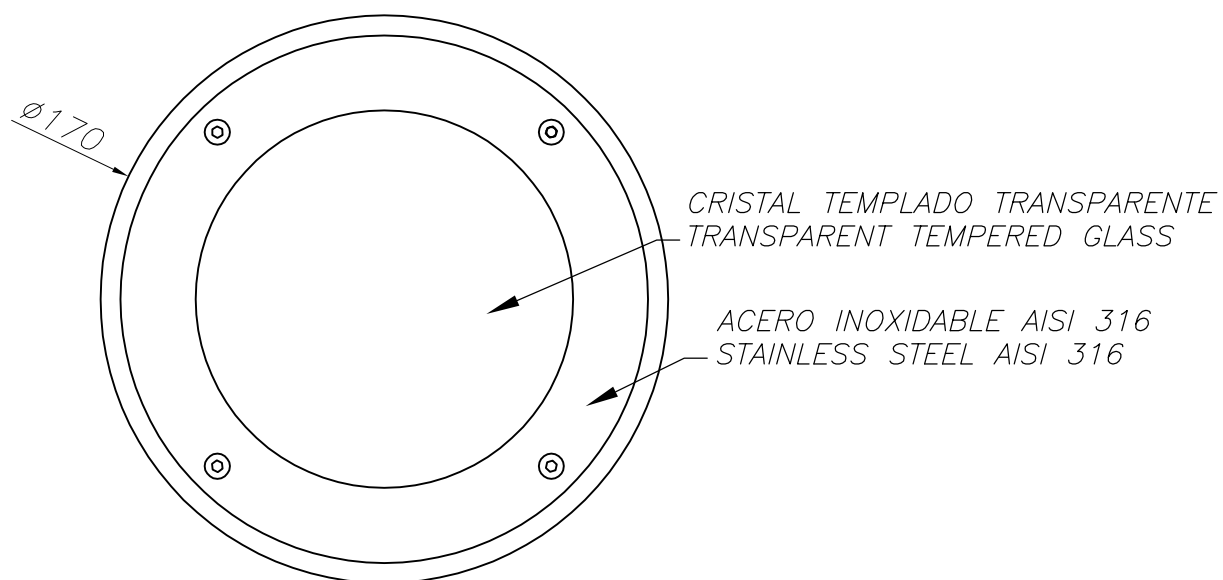
CAJA DE EMPOTRAR FLUSH FITTING BOX
