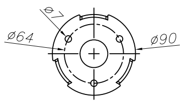
PLANTILLA DE INSTALACIÓN INSTALLATION TEMPLATE
