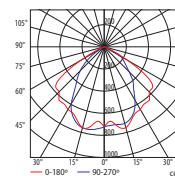
PL-R GR14q-1 2X17W
