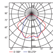
TC-DEL G24q-2 2X18W
