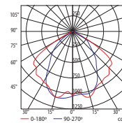
TC-TEL GX24q-3+q-4 2X26W
