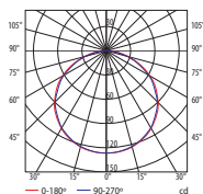
91-4671 LED Blanco cálido / Warm white
