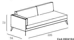
DIVANO 3 POSTI LATERALE | 3-SEATER SIDE SOFA Rappresentato SX | L/h shown
