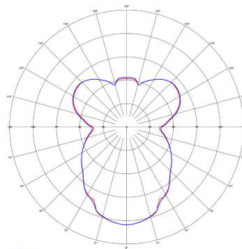
DIAGRAMMA POLARE (cd/klm)
