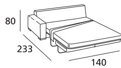
Laterale letto 3 posti da 190 Dx/Sx 3 seater Rh/Lh side elem. cm 190
