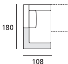
Angolo terminale da 180x108 Dx/Sx Rh or lh corner end element cm 180x108
