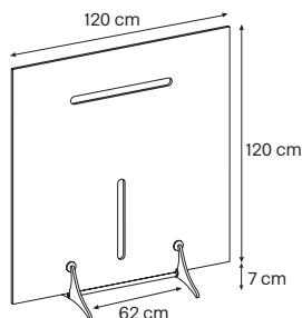
cm 120 x h 127
