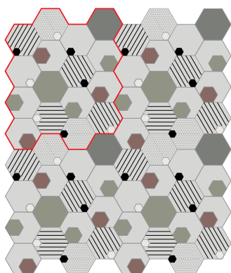
Schema di posa - 6 colori Formati (7): H1/H2/H3/H4/H5/HL/HP
