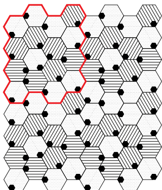
Schema di posa - 7 formati
