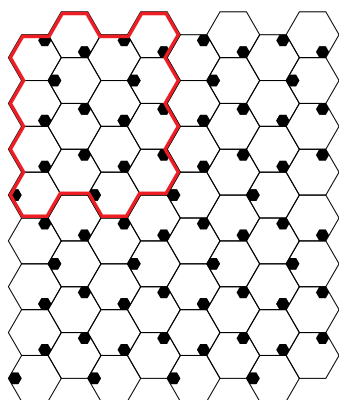
Schema di posa - 2 formati
