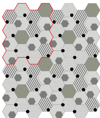
Schema di posa - 4 colori Formati (6): H1/H2/H3/H5/HL/HP
